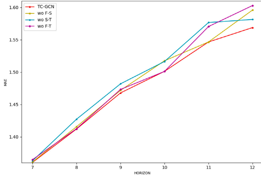
(b) PEMS-BAY dataset
