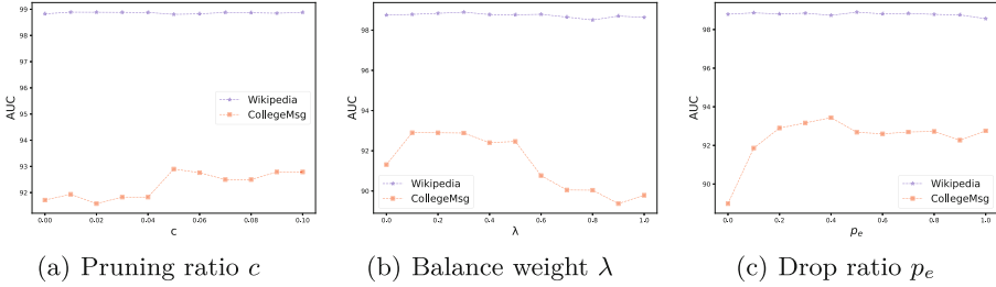
Fig. 3. Parameter Sensitivity.
